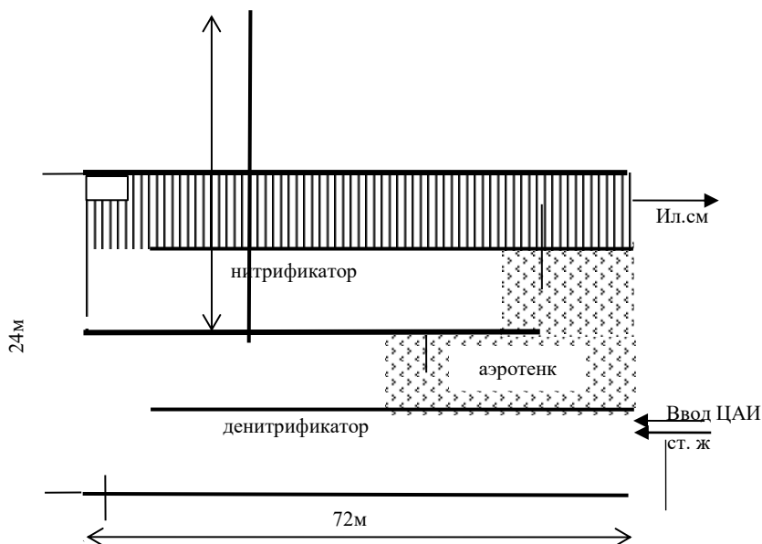
Рис.2. Распределение объемов сооружения между денитрификатором, аэротенком и нитрификатором.
