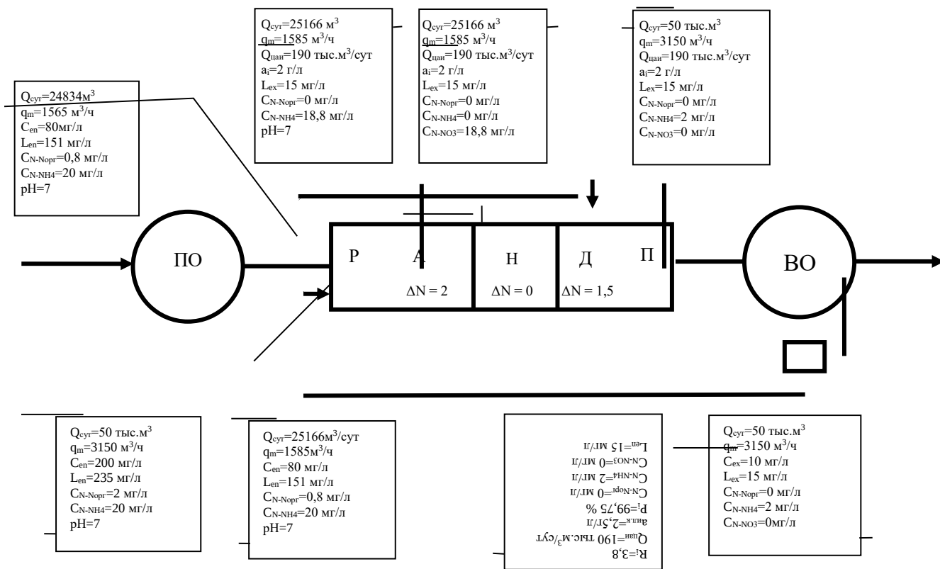
Рис.7. Балансовая схема к примеру расчета по схеме «в»
