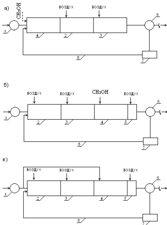
Рис.1. Возможные схемы удаления из сточной жидкости азота методом нитрификации-денитрификации. 1-первичный отстойник; 2-аэротенк; 3-нитрификатор; 4-денитрификатор; 5-постаэратор; 6-вторичный отстойник; 7-насосная станция циркулирующего активного ила; 8-циркулирующий активный ил.
