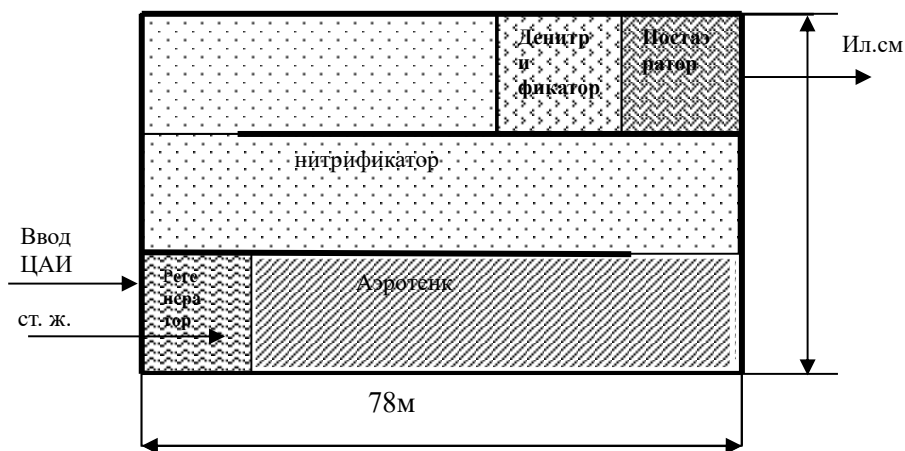
Рис.4. Распределение объема сооружения между аэротенком с регенератором, нитрификатором, денитрификатором и постаэротенком.
