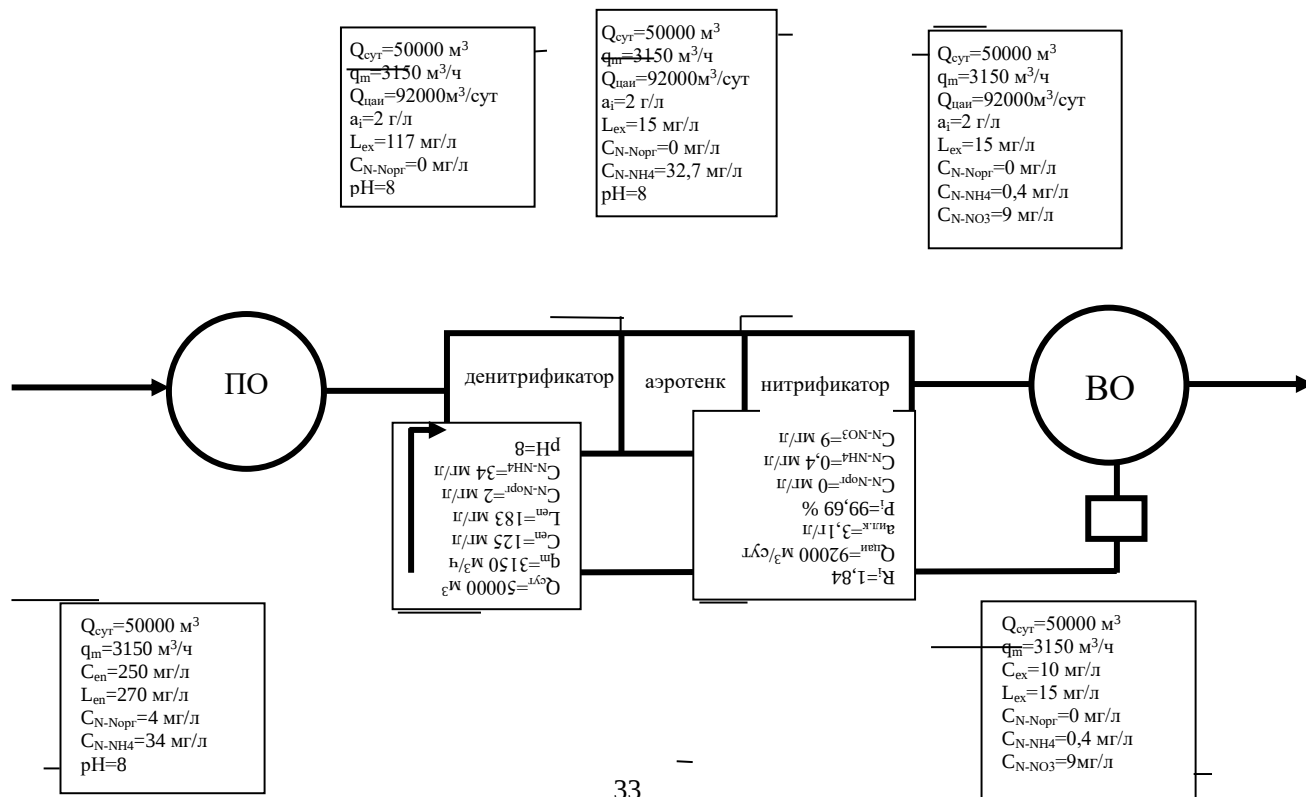
Рис.3. Балансовая схема к примеру расчета по схеме «а»
